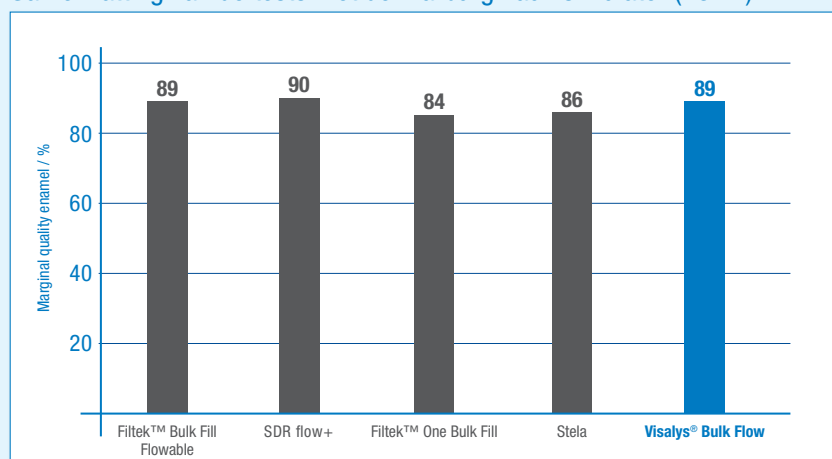
Samenvatting van de tests met de Marburg kauwsimulator (TCML)*
